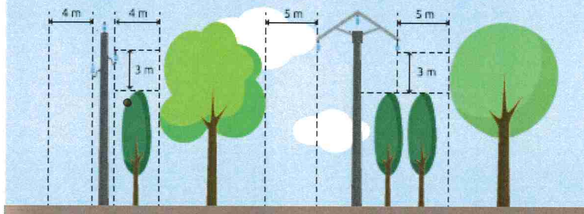
Isolateurs rigides
